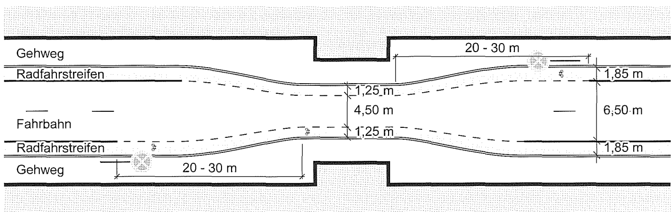
Bild 16: Übergang eines Radfahrstreifens in einen Schutzstreifen im Bereich einer Engstelle
