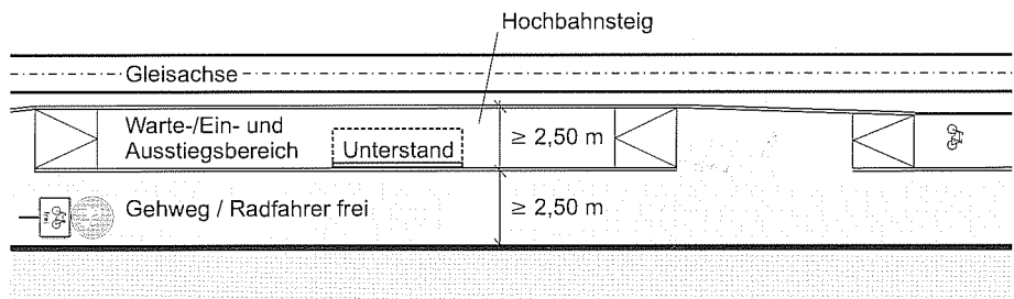
Bild 29: Umfahrung einer Haltestelle mit Hochbahnsteig
