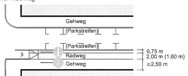
baulicher Radweg
